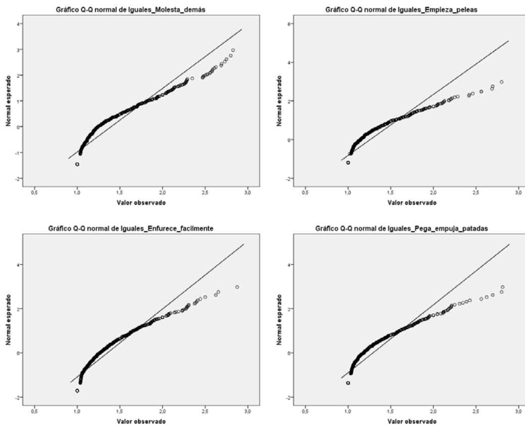
Gráfico 4 Gráficos Q-Q de los criterios de la calificación de agresividad
