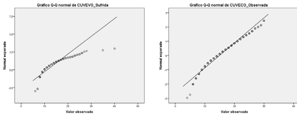
Gráfico 2 Gráficos Q-Q de los factores del CUVECO
